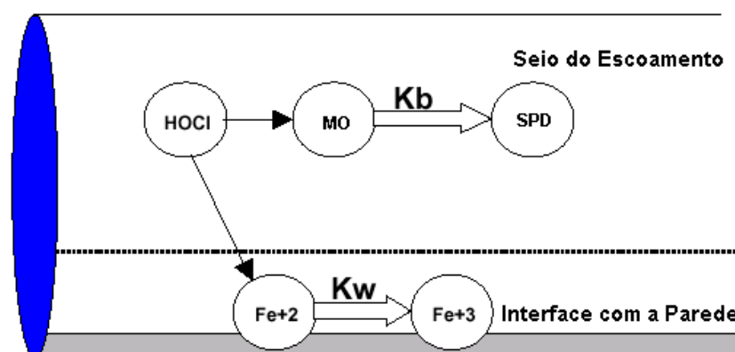
Figura 3.6 Zonas de Reacção no Interior de uma Tubagem
