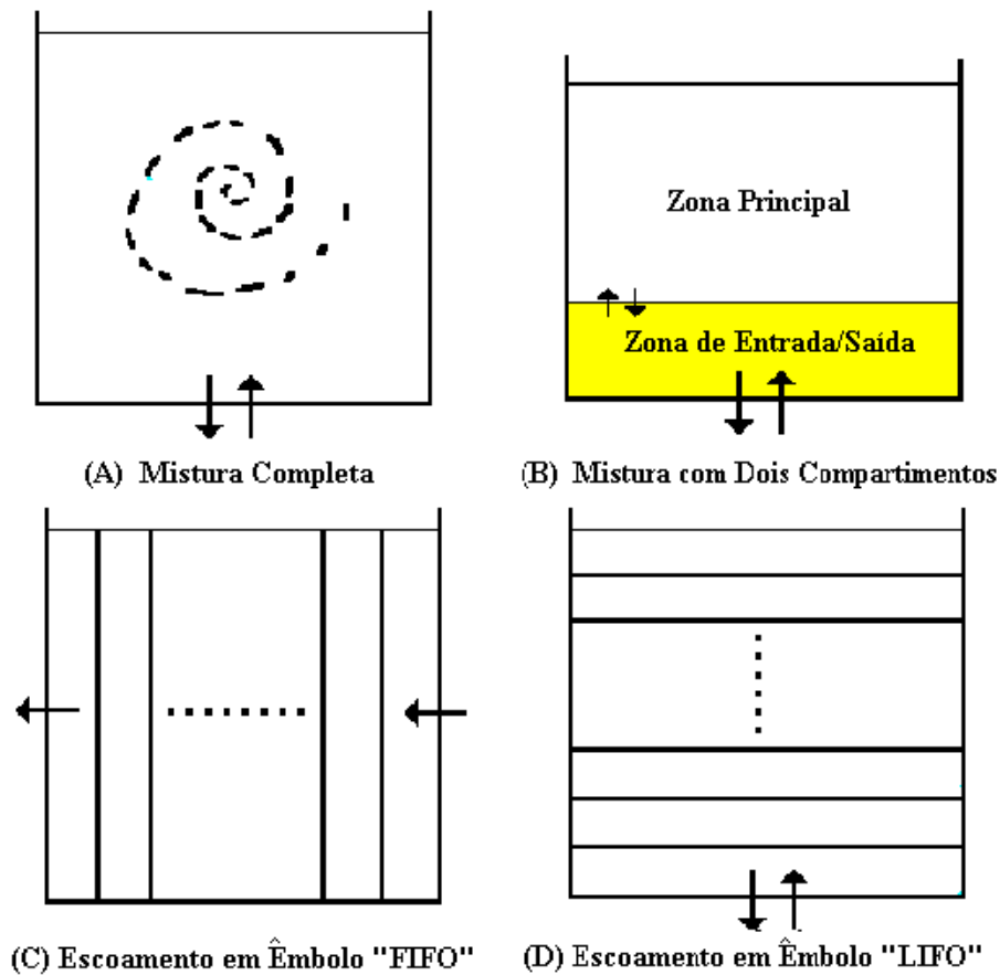
Figura 3.5 Modelos de Mistura em Reservatórios de Nível Variável
