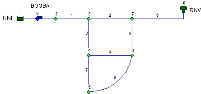
Figura 2.1 Representação da Rede Exemplo no EPANET
