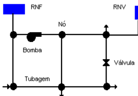
Figura 3.1 Componentes Físicos de um Sistema de Distribuição de Água
