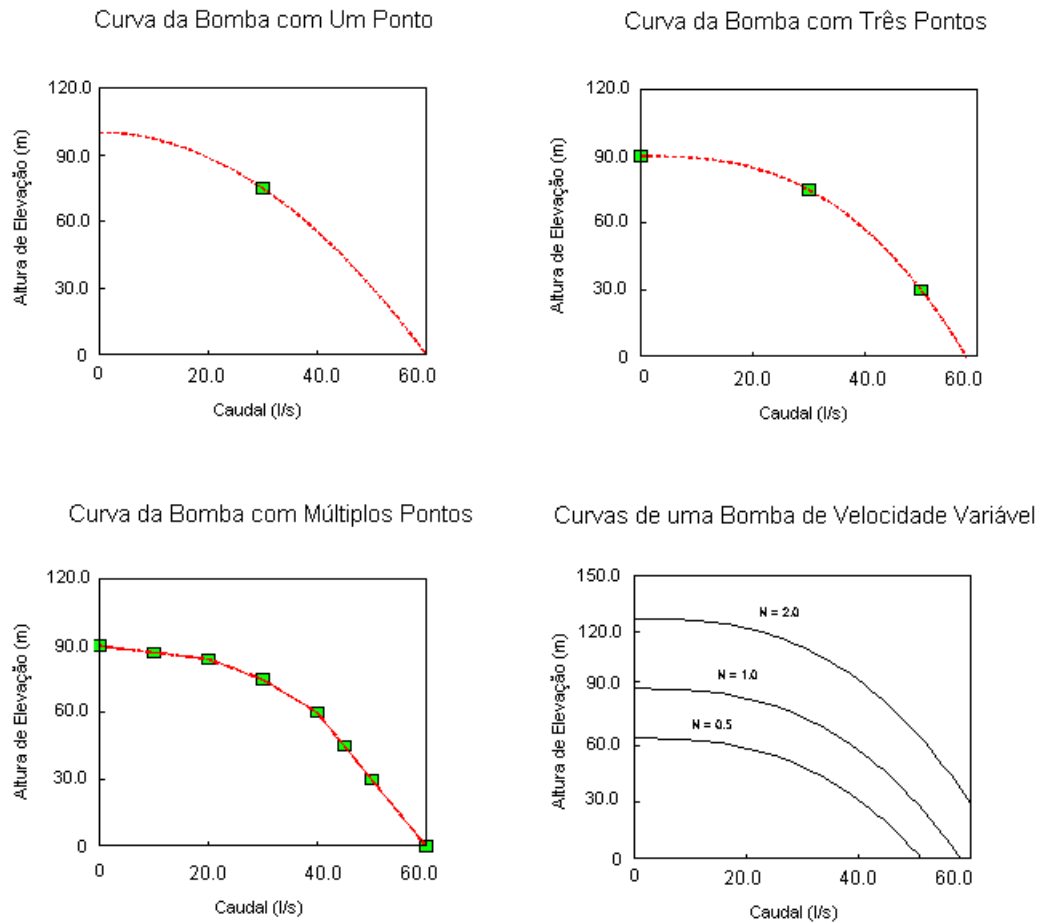
Figura 3.2 Exemplo de curvas de bombas
