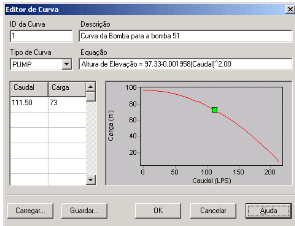
Figura 2.6 Editor de Curva
