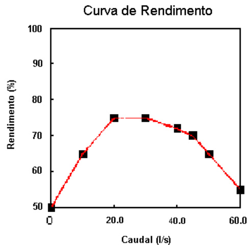
Figura 3.3 Curva de Rendimento da Bomba
