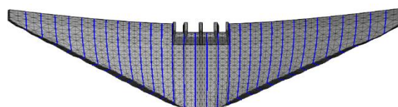
Fig. 8 - Vista de jusante do modelo numérico da barragem do Baixo Sabor com representação dos blocos limitados pelas juntas de contração
