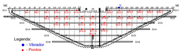
Fig. 6 - Plano de colocação da aparelhagem utilizada durante o ensaio de vibração forçada
