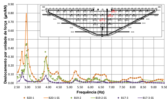
Fig. 7 -Funções de resposta de força para deslocamento. Comparação entre os resultados os ensaios realizados por varrimentos discreto e contínuo (SineSweep SS).
