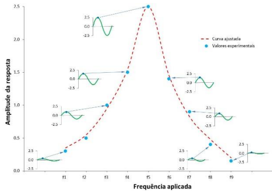
Fig. 1 - Função de transferência em frequência da resposta de um ponto da estrutura obtida num ensaio de vibração forçada por varrimento discreto de frequência
