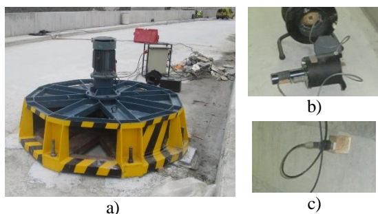
Fig. 5 - Pormenor de colocação do: a) vibrador de massa excêntrica, b) transdutor de velocidade e c) acelerômetro
