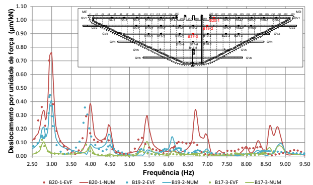
Fig. 9 - Comparação das funções de resposta em frequência obtidas a partir dos resultados do ensaio de vibração forçada (EVF) e do modelo numérico (NUM).
