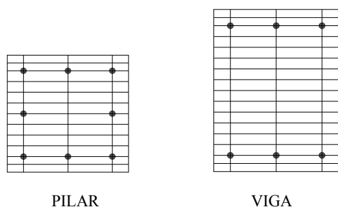
Fig 24 – Discretização em fibras (Pilar e Viga).
