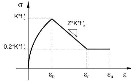
Fig 23 – Modelo de Kent e Park (betão).
