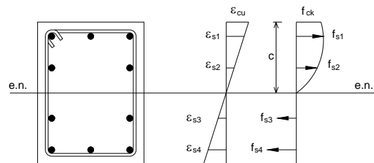
Fig 8 – Base para a determinação da cedência em barra de betão armado.
