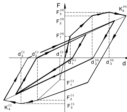
Fig 19 – Curva força-deslocamento (Takeda tetralinear).
