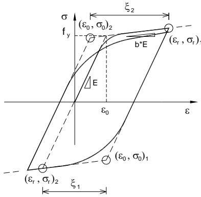
Fig 22 – Modelo de Magenotto-Pinto (aço).
