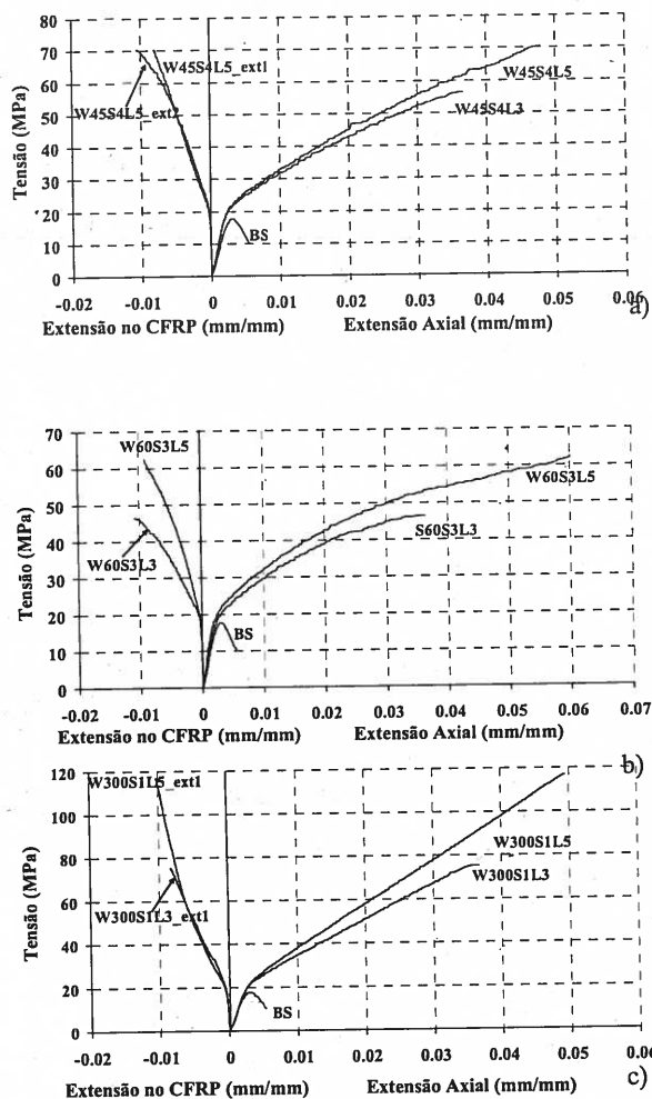
Fig. 7- Relação tensão versus extensão axial e extensão no CFRP nas séries do grupo C16S300.
