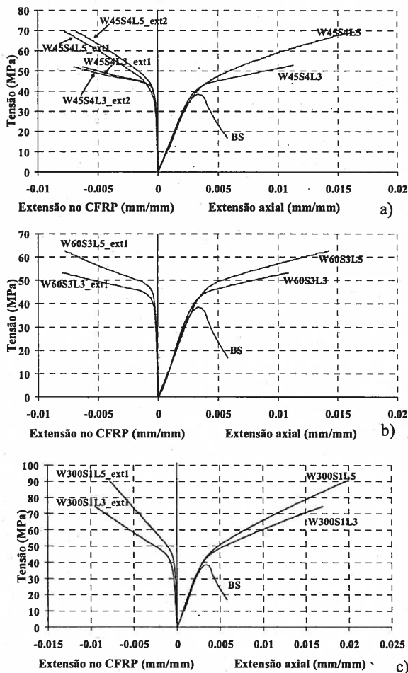
Fig.5- Relação tensão versus extensão axial e extensão no CFRP nas séries do grupo C23S200.
