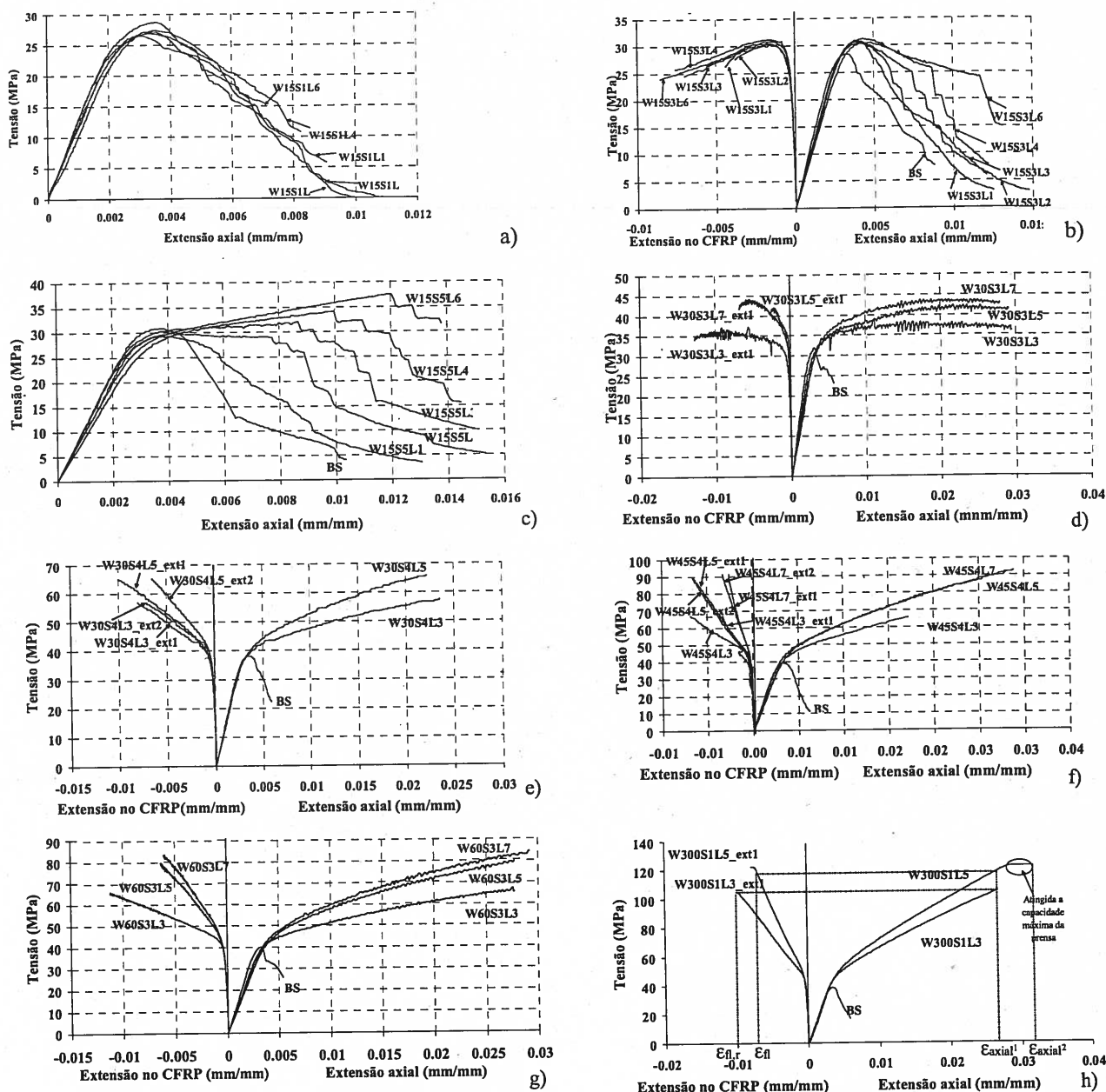
Fig. 4 – Relação tensão versus extensão axial e extensão no CFRP nas séries do grupo C23S300
