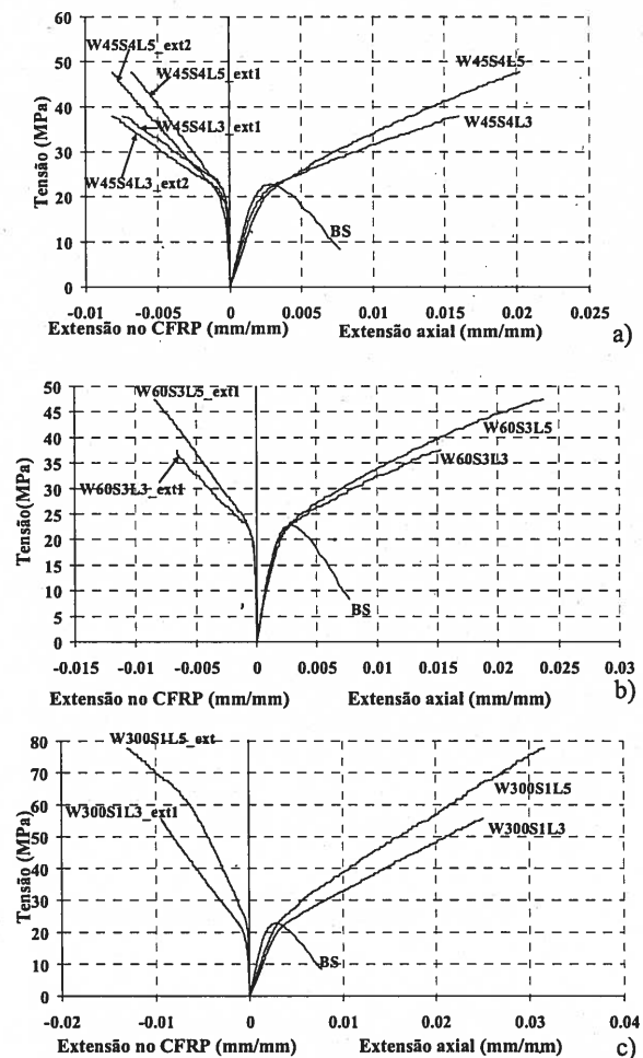
Fig.6 – Relação tensão versus extensão axial e extensão no CFRP nas séries do grupo C16S200.
